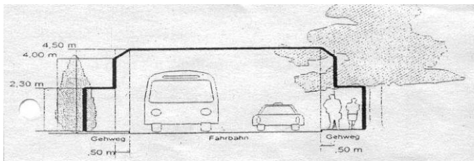
Abb.: Das Lichttraumprofil an öffentlichen Straßen und Gehwegen
