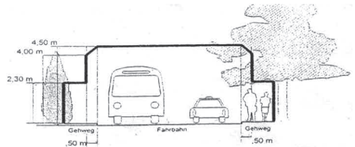
Abb.: Das Lichtraumprofil an öffentlichen Straßen und Gehwegen
